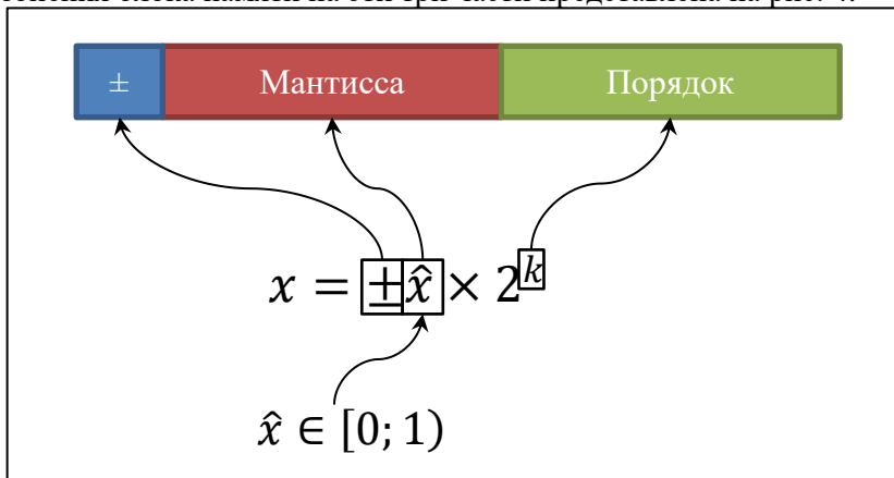
Рис. 4. Представление числа с плавающей запятой в памяти компьютера
