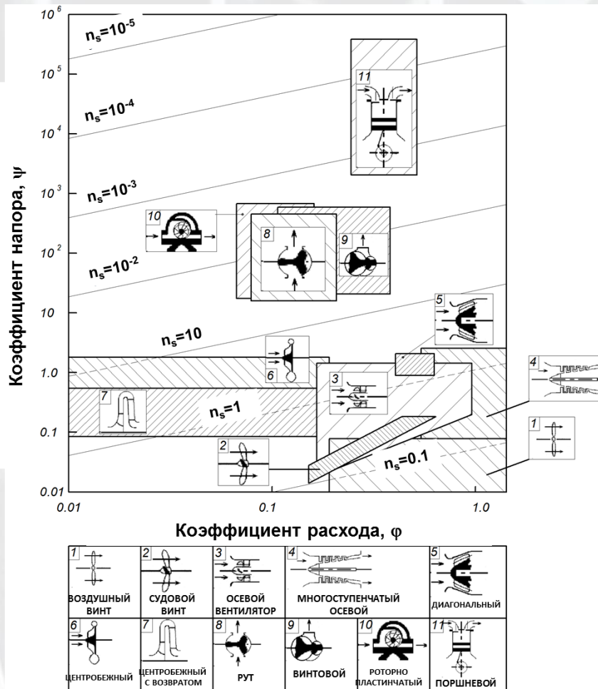
Рисунок 1.3 - Области применени я разных сжимающи х устройств [9]
