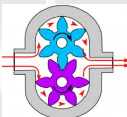
Компрессор "Рут"
